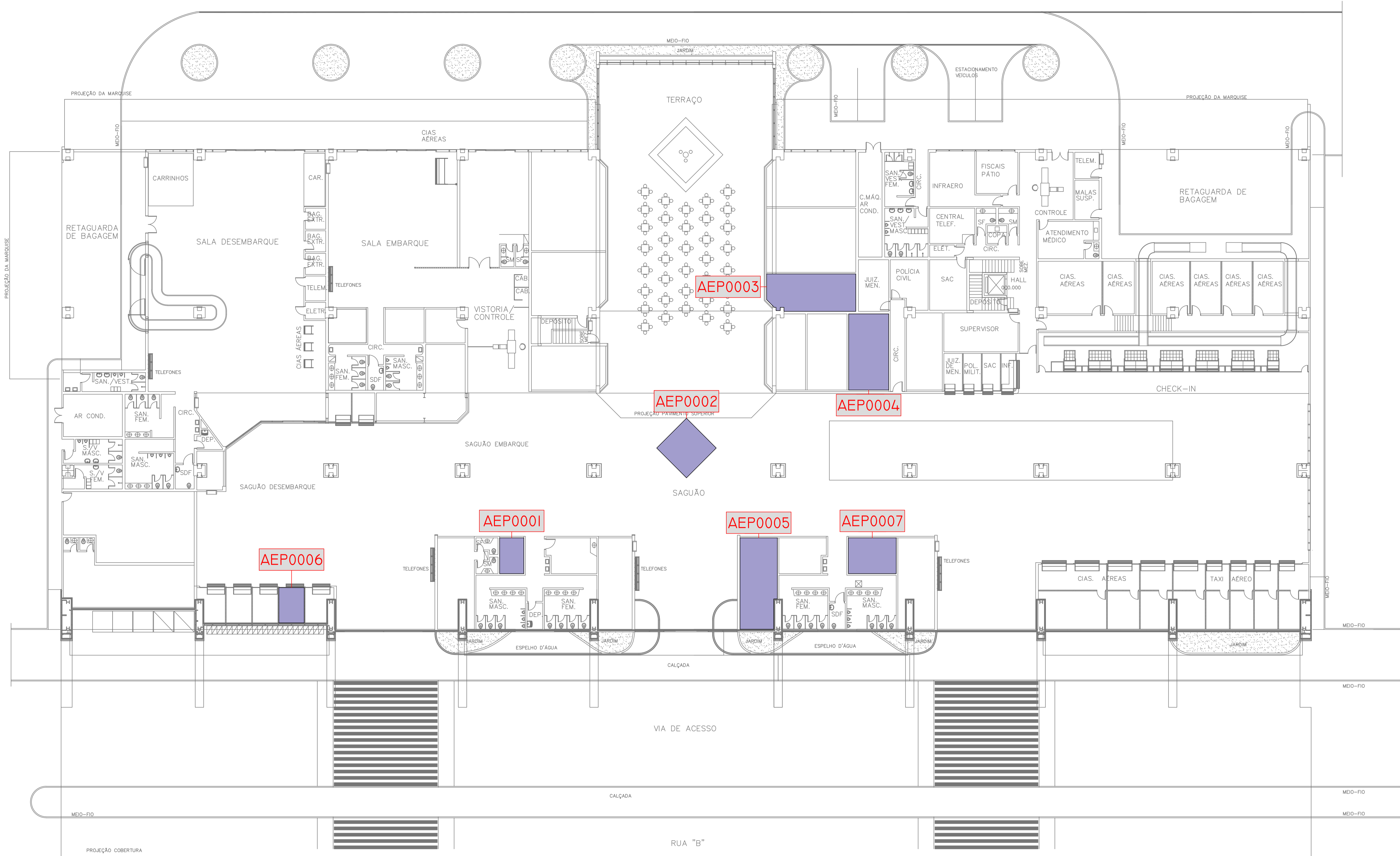
PLANTA BAIXA - PAVIMENTO TÉRREO ESCALA 1:175
